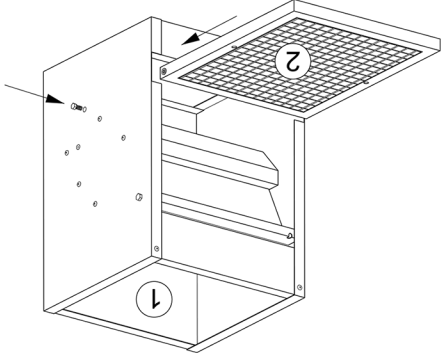
Fig.1 Entfernen Sie die Schrauben von der Trittklappe. Positionieren Sie Die Trittklappe, indem Sie seine Löcher mit denen an den Seiten abstimmen. Setzen Sie die Schrauben ein und ziehen Sie sie fest.
