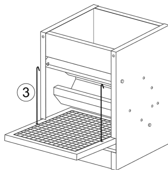
Fig.2 Colocar ganchos con la posición según figura.
