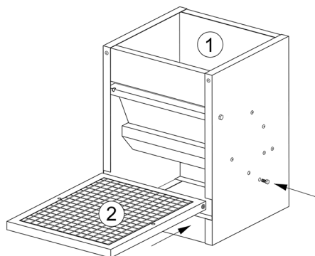
Fig.1 Quitar los tornillos de la paradera. Posicionar la paradera haciendo coincidir los orificios de esta con los de los laterales. Insertar y apretar los tornillos.
