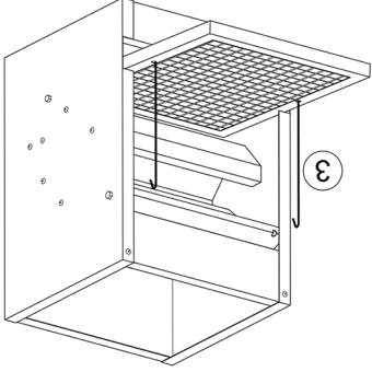
Fig.2 Positionieren Sie die Haken an der in der Abbildung gezeigten Position.
