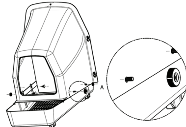
FIGURA 2 Use los tornillos y las tuercas de plástico para fijar la cubeta al ponedero.
