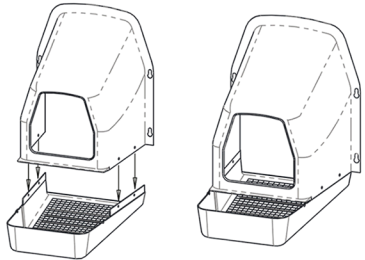
FIGURA 1 Alinee los agujeros de la cubeta y el ponedero como se muestra.
