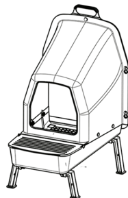
FIGURA 4 Alinee la tapa trasera negra con los agujeros como se muestra. Inserte un tornillo de plástico en cada orificio y utilice las tuercas de mariposa para asegurar la tapa al ponedero.
